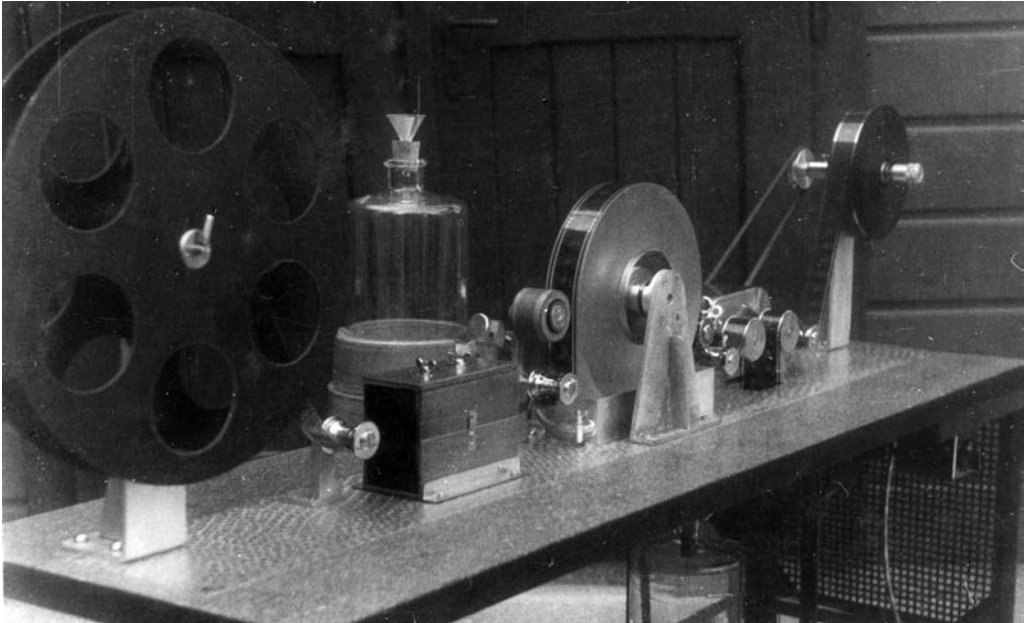
Saját tervezésű filmpolirozó berendezése, amely még a '80-as években is üzemben volt a budapesti filmlaboratóriumban (az eljárás célja a régi elhasználódott kópiák karctalanítása volt, amit 70%-os sikerrel el lehetett végezni ezzel a berendezéssel)
